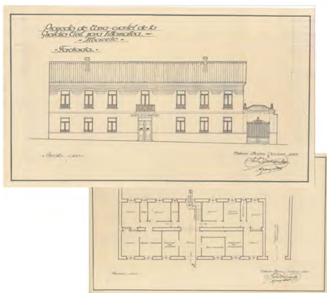
Proyecto de obras para reforma y construcción de casa cuartel de la Guardia Civil en Villamalea. 1930.
