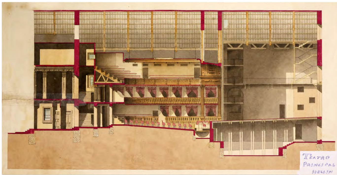
Sección del desaparecido Teatro Principal (1890-1892), obra del arquitecto Justo Millán.
