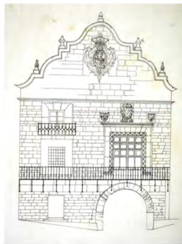
Dibujo de la fachada principal y lateral del edificio del Ayuntamiento realizado en papel vegetal.
