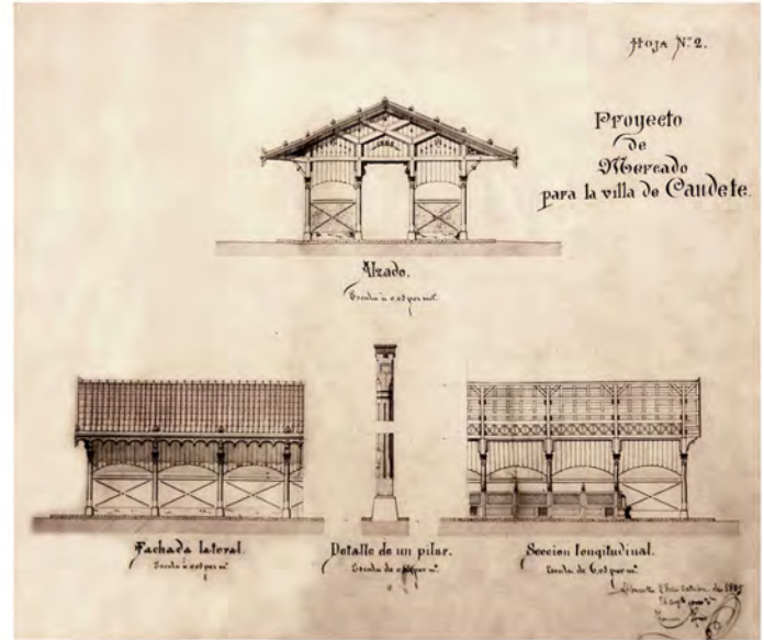
AMC. Proyecto de obras del mercado municipal. Arquitecto Tomás Rico, 1885.
