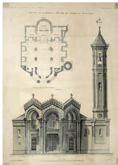
Planos y dibujo de la ermita del Rosario de Hellín (1875-1877).
